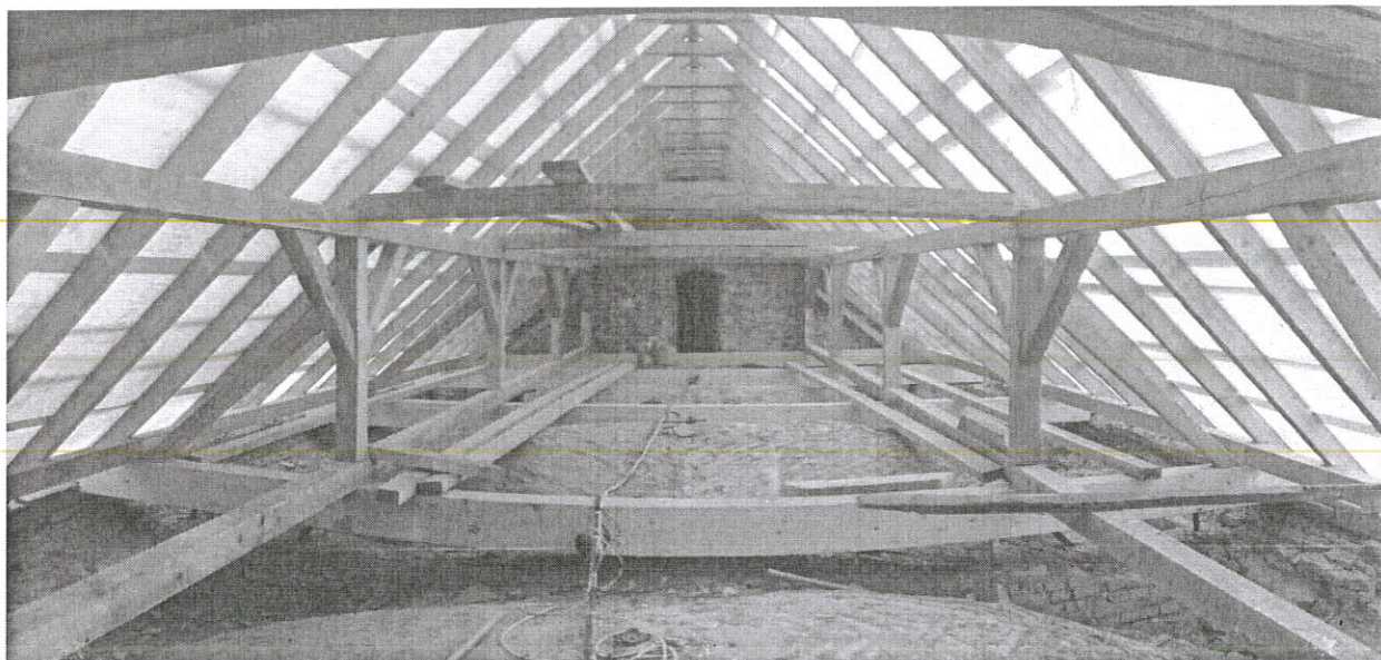
Új faszerkezet a tetőtérben
