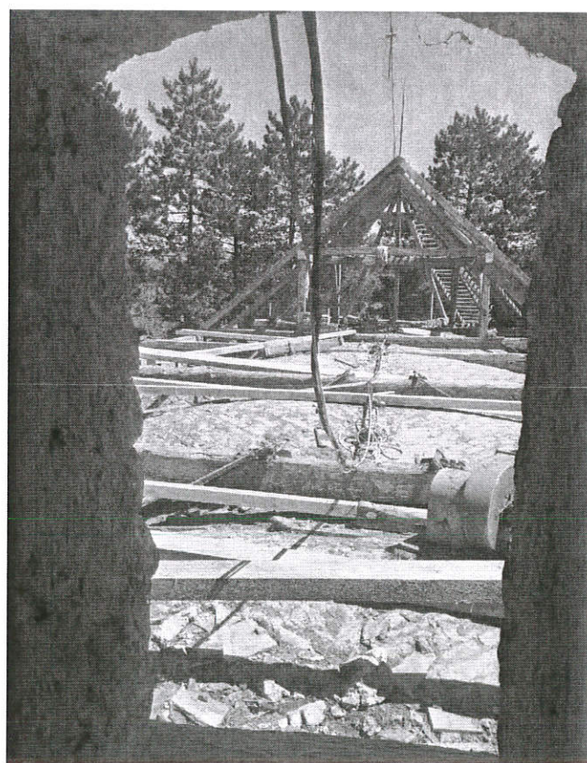
A tetőszerkezet elbontását követően
